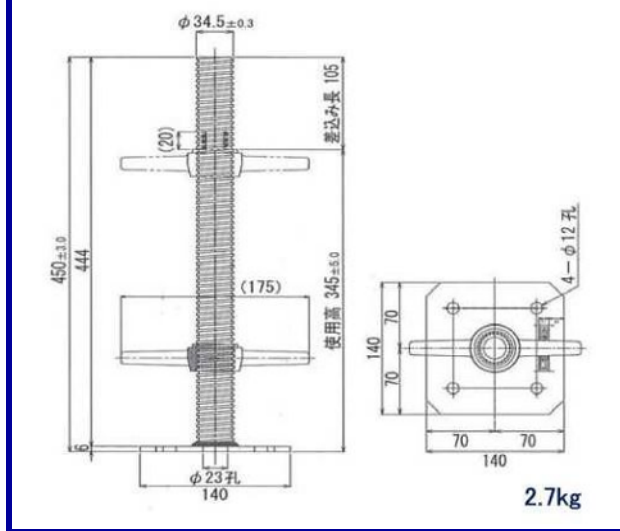
中空ジャッキベース
