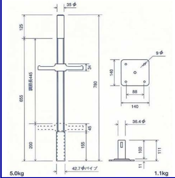
棒ジャッキ・ベース
