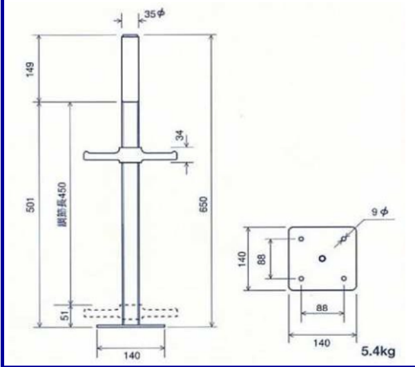
ロングジャッキベース
