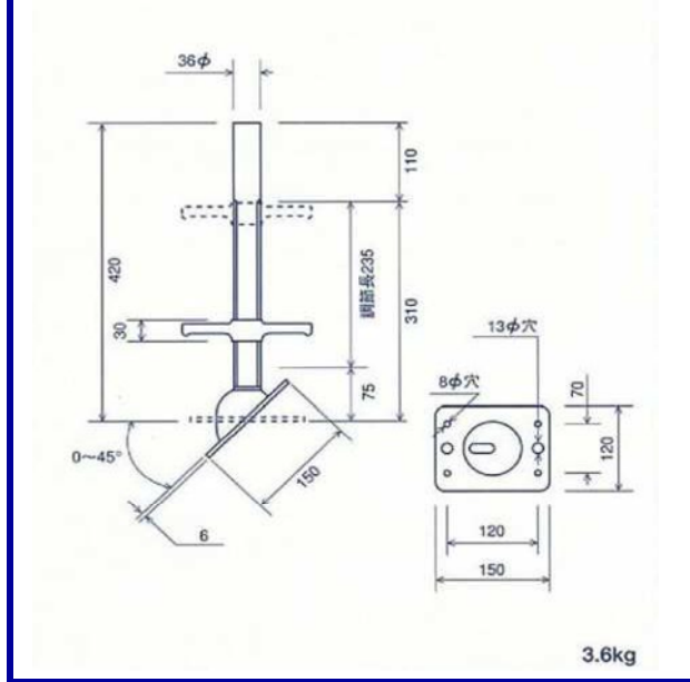
ピポットジャッキ
