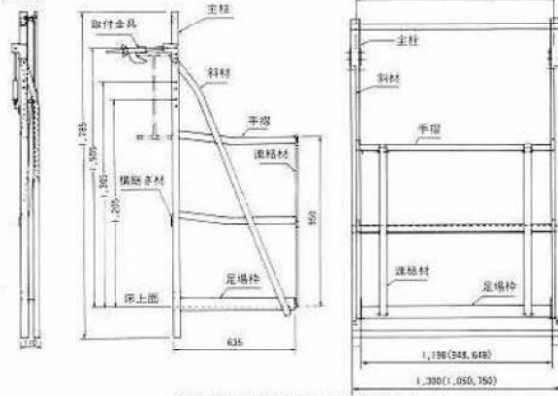
※取付金具および横置き材の高さは、3段階調節が可能です。
